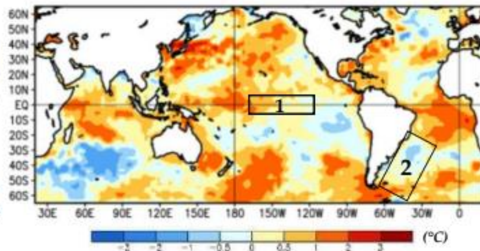
Fig. 17: Promedio semanal de las anomalías de temperaturas ( ^{\circ}\text{C} ) de la superficie del mar desde el 12/01/20 hasta el 08/02/2020.
