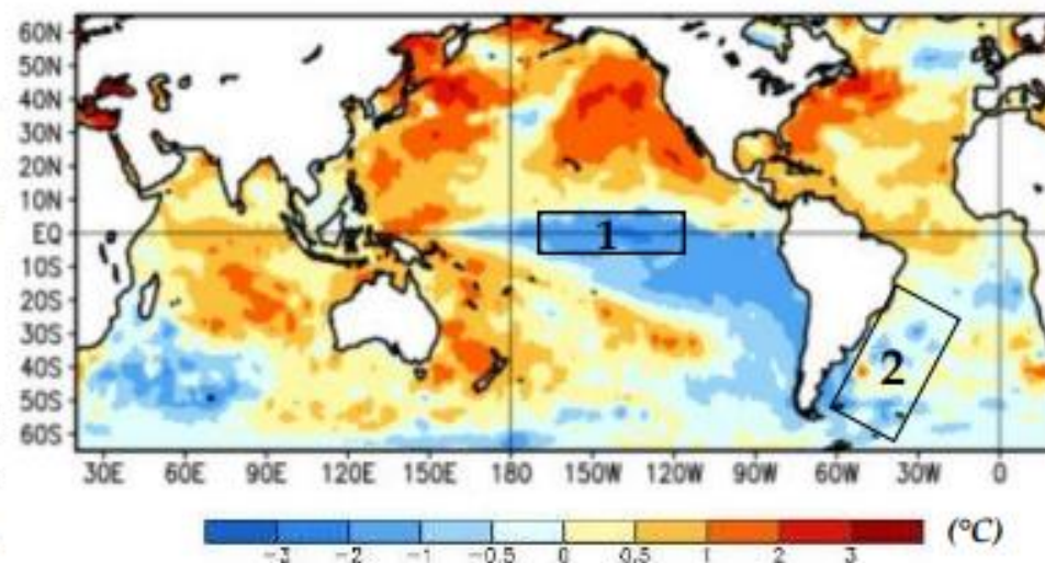
Fig. 39: Promedio semanal de las anomalías de temperatura ( ^{\circ}\text{C} ) de la superficie del mar desde el 11/10/2020 hasta el 04/11/2020.
