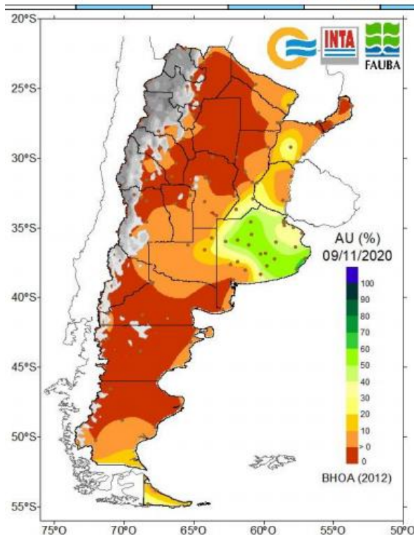
Fig. 25: Agua útil (%) en el perfil del suelo al 09/11/2020.
