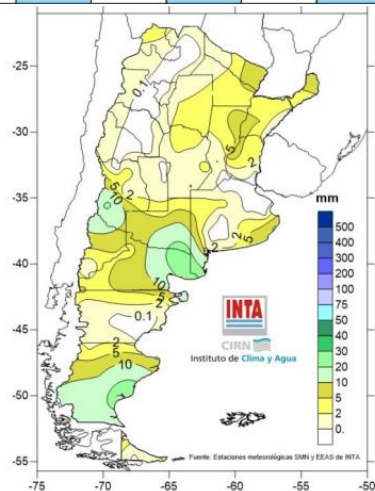
Fig. 24: Precipitación (mm) observada entre el 02 y el 09 de Noviembre de 2020 (9:00 hs.).
