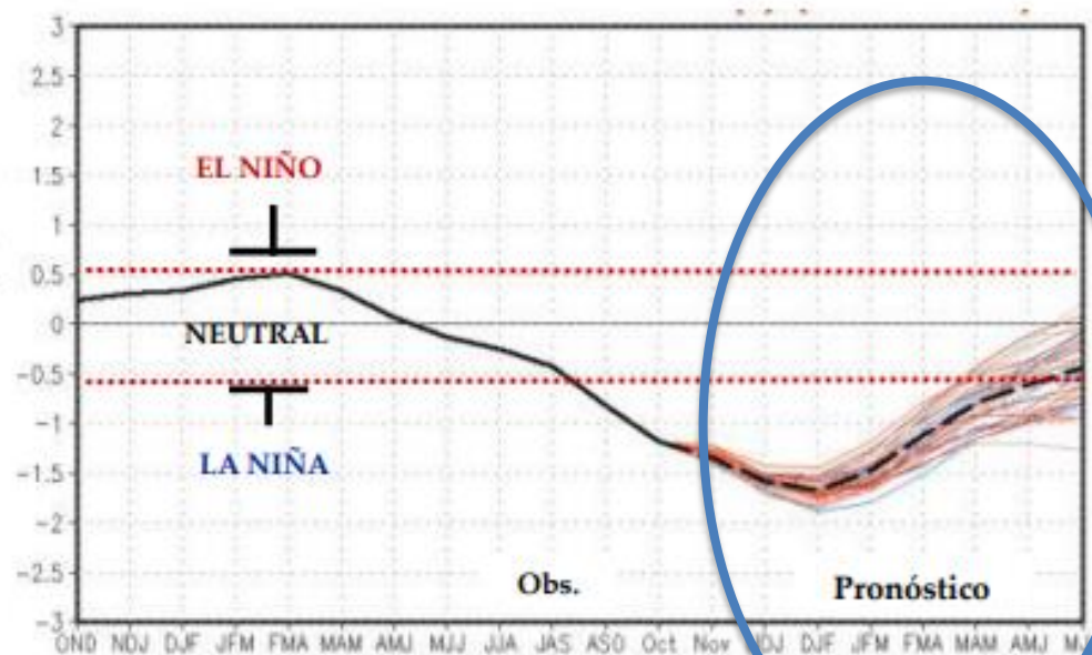
Fig. 40: Evolución de la anomalía trimestral observada y pronóstico de la temperatura de la superficie del mar (°C) en el Océano Pacífico Ecuatorial en la región Niño 3.4 (actualizado al 09/11/2020).
