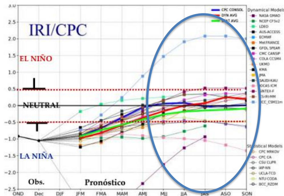
Fig. 20: : Evolución de la anomalía trimestral observada y pronóstico de la temperatura de la superficie del mar (°C) en el Océano Pacífico Ecuatorial en la región Niño 3.4 (actualizado al 19/01/2022).
