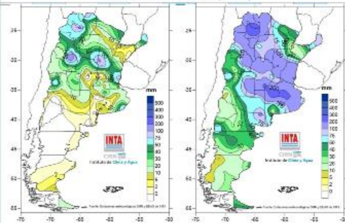
Fig. 01: Precipitación (mm) observada entre el 24 al 31 de Enero de 2022 (9:00 hs.).
