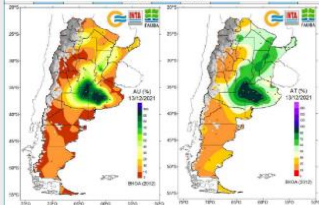
Fig. 04: Agua útil (%) en el perfil del suelo.
