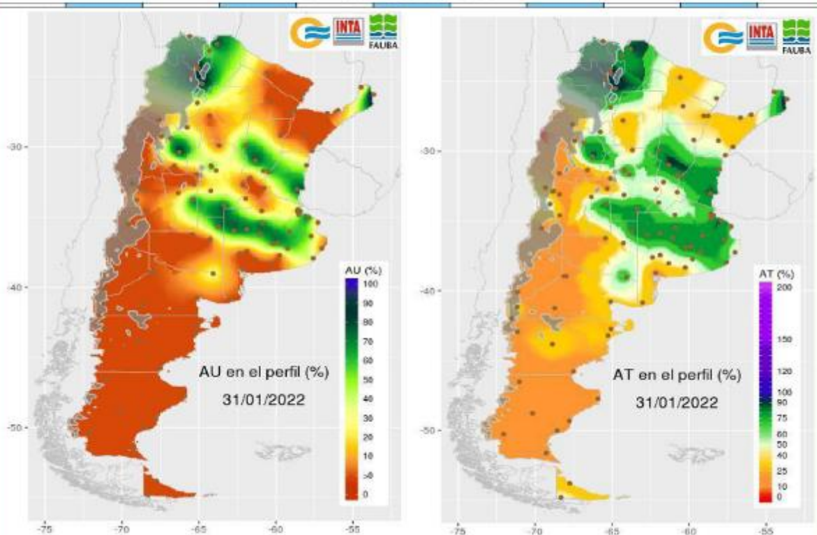
Fig. 04: Agua Total (%) en el perfil del suelo.
