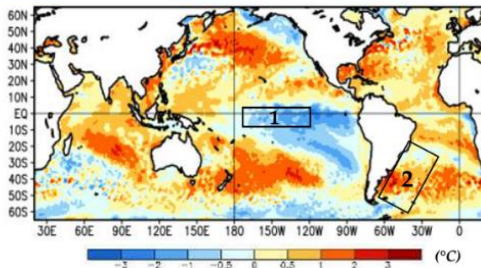
Fig. 19: Promedio de las anomalías de temperatura ( ^{\circ}\text{C} ) de la superficie del mar desde el 2/1/2022 hasta el 29/01/2022.
