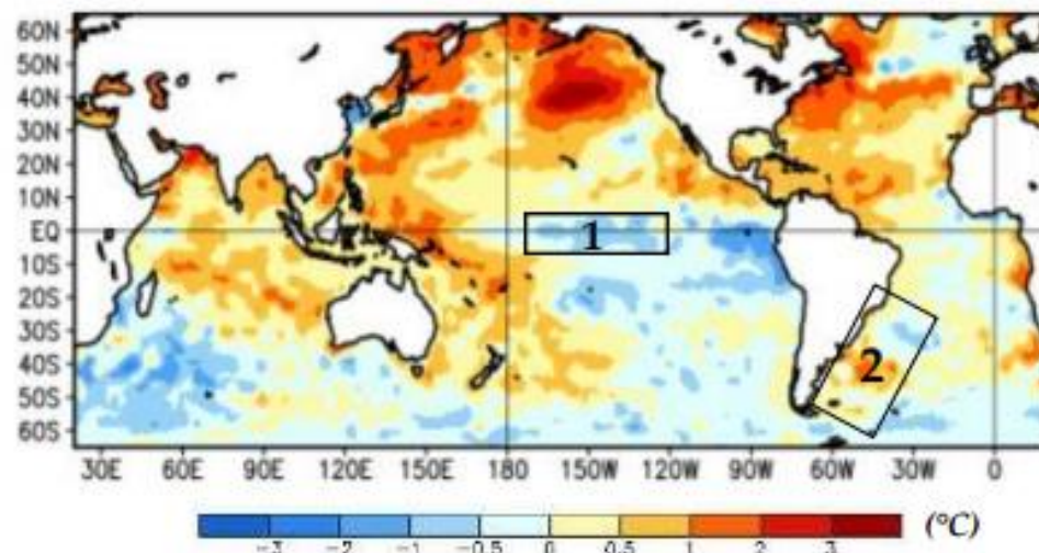
Fig. 17: Promedio semanal de las anomalías de temperaturas ( ^{\circ}\text{C} ) de la superficie del mar desde el 12/07/2020 hasta el 08/08/2020.
