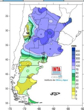
Fig. 01: Precipitación (mm) observada durante el mes de Enero de 2021.
