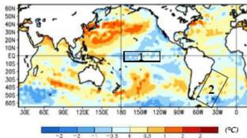
Fig. 18: Promedio semanal de las anomalías de temperatura ( ^{\circ}\text{C} ) de la superficie del mar desde el 07/03/2021 hasta el 03/04/2021.
