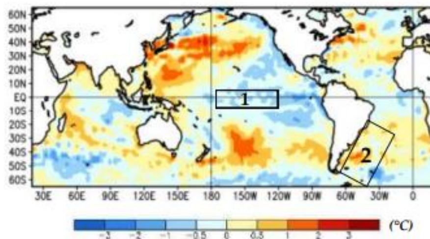
Fig. 19: Promedio semanal de las anomalías de temperatura ( ^{\circ}\text{C} ) de la superficie del mar desde el 21/03/2021 hasta el 17/04/2021.
