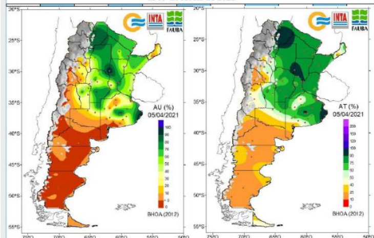
Fig. 03: Agua útil (%) en el perfil del suelo al 05/04/2021.
