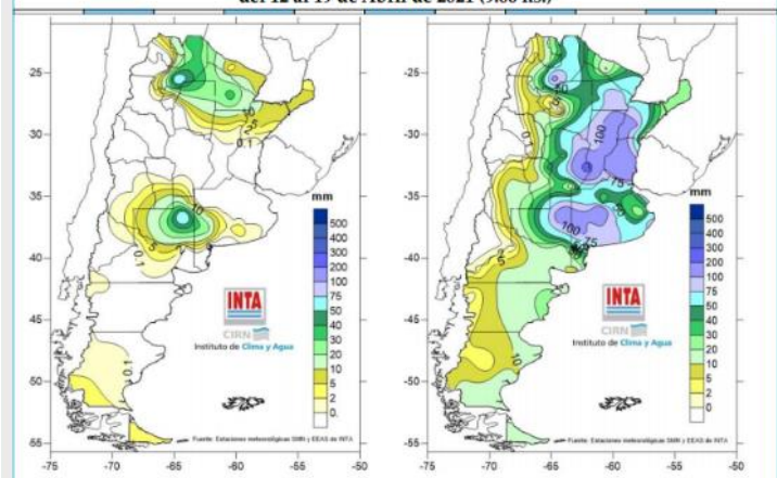
Fig. 01: Precipitación (mm) observada entre el 12 y el 19 de Abril de 2021 (9:00 hs.).
