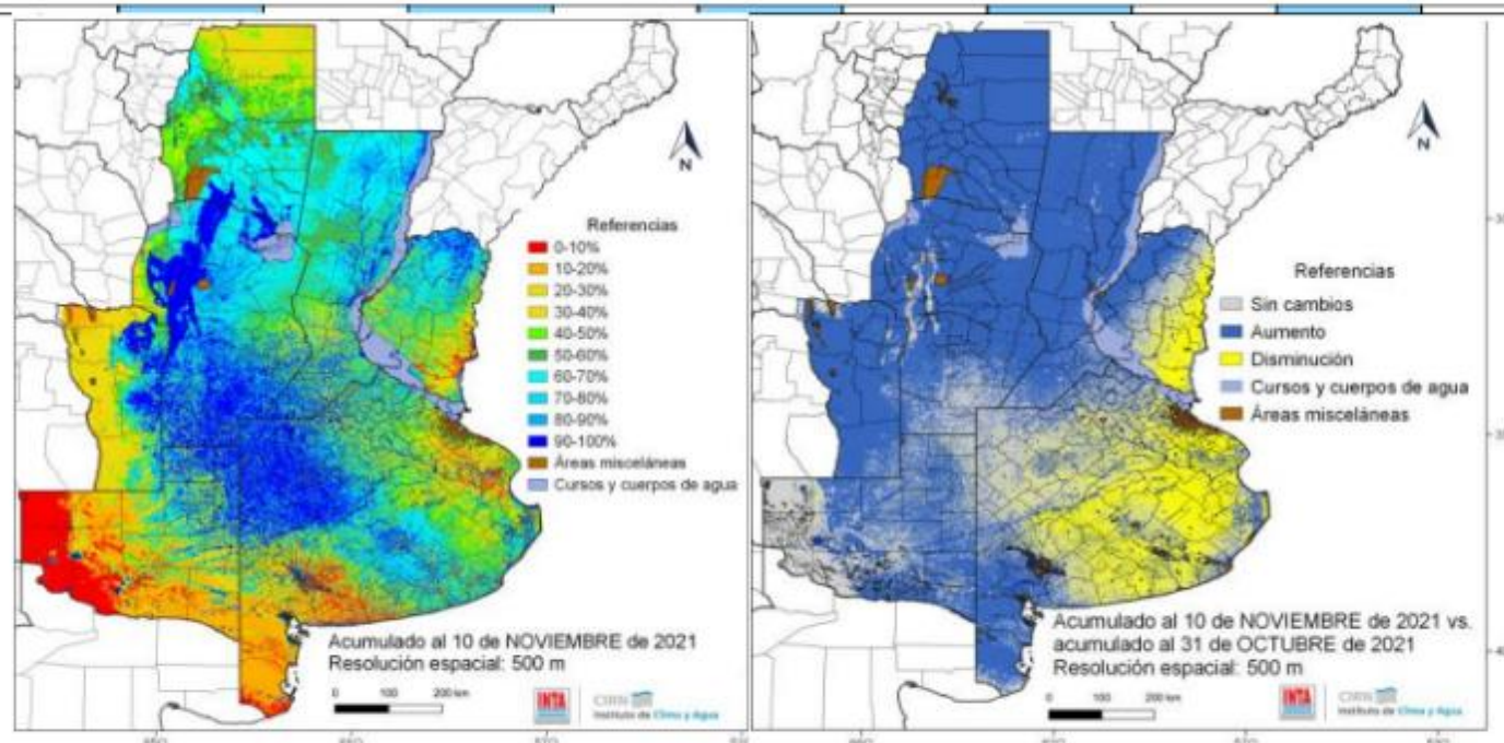
Fig. 03: Agua en el suelo (%) hasta 1m (izquierda) y su variación con respecto a la década anterior (derecha).
