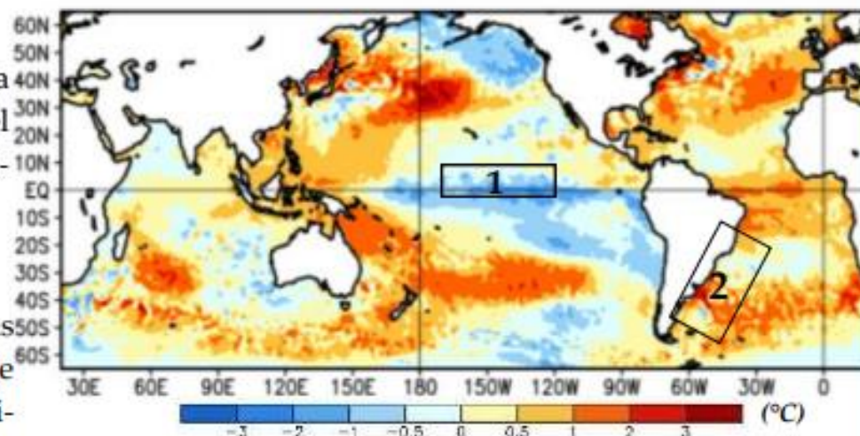
Fig. 21: Promedio de las anomalías de temperatura ( ^{\circ}\text{C} ) de la superficie del mar desde el 24/10/2021 hasta el 20/11/2021.
