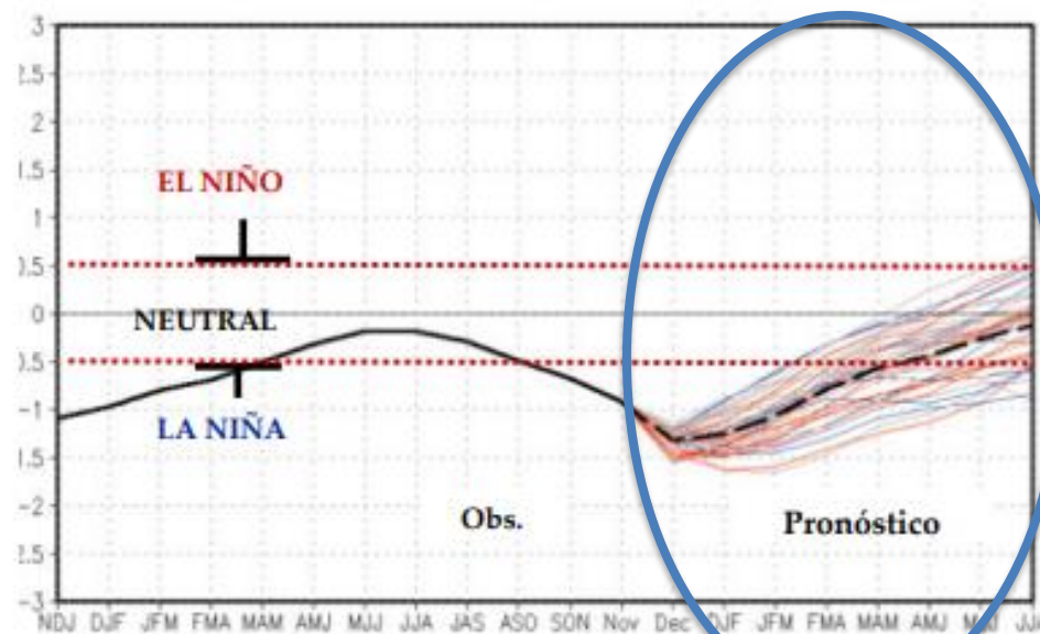
Fig. 22: Evolución de la anomalía trimestral observada y pronóstico de la temperatura de la superficie del mar (°C) en el Océano Pacífico Ecuatorial en la región Niño 3.4 (actualizado al 22/11/2021).
