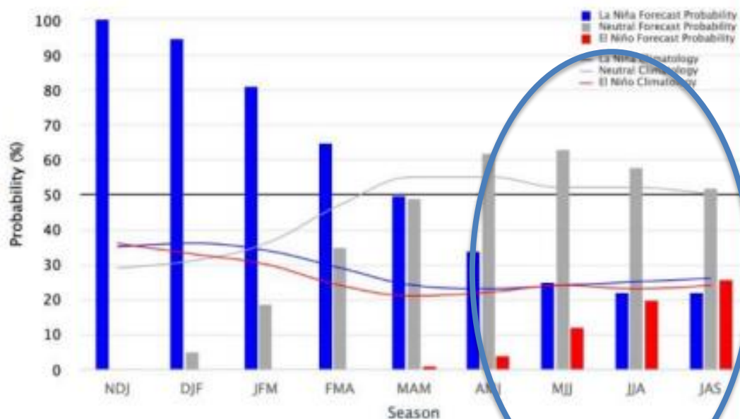
Fig. 18: Probabilidad de ocurrencia de cada fase ENSO, basada en el resultado de modelos de simulación tanto dinámicos como estadísticos (actualizado al 09/12/2021).
