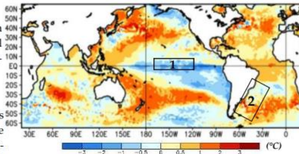
Fig. 17: Promedio de las anomalías de temperatura ( ^{\circ}\text{C} ) de la superficie del mar desde el 14/11/2021 hasta el 11/12/2021.
