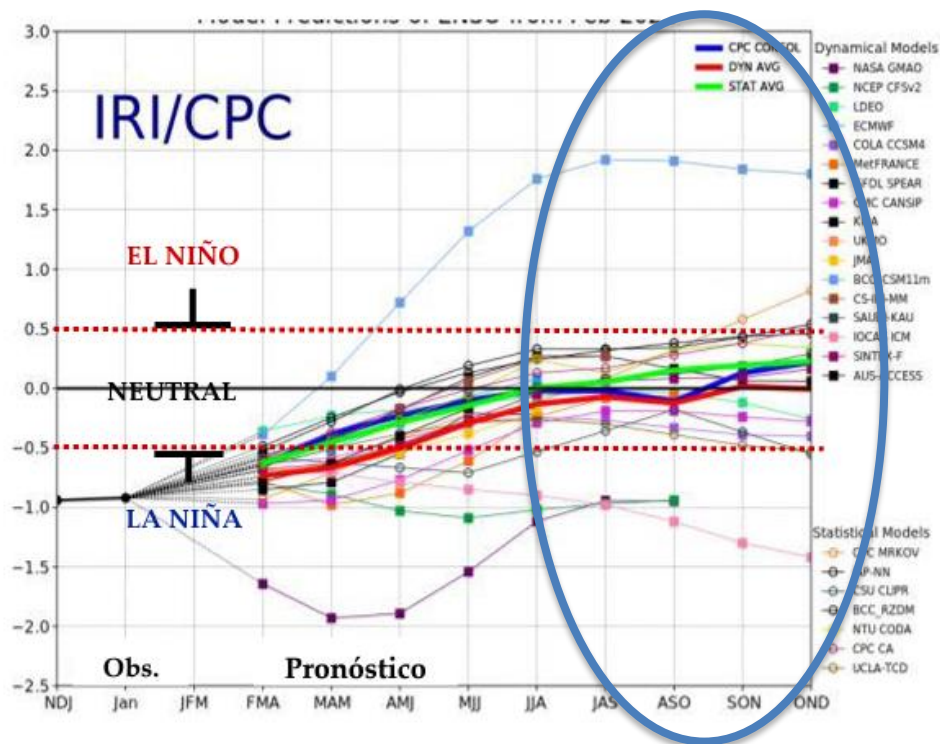
Fig. 22: Evolución de la anomalía trimestral observada y pronóstico de la temperatura de la superficie del mar (°C) en el Océano Pacífico Ecuatorial en la región Niño 3.4 (actualizado al 18/02/2022).
