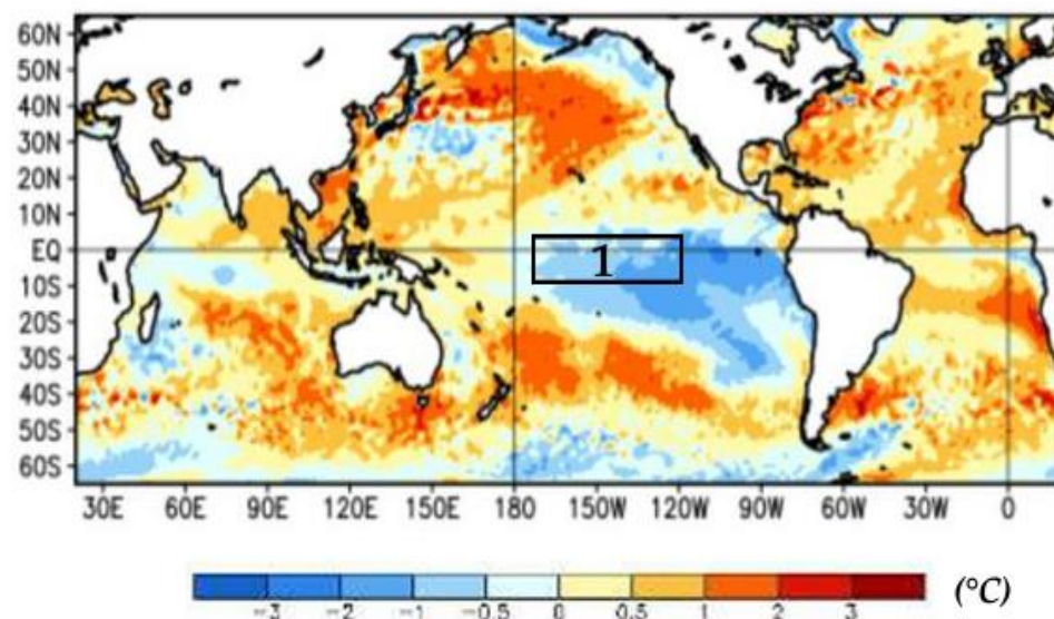
Fig. 21: Promedio de las anomalías de temperatura ( ^{\circ}\text{C} ) de la superficie del mar desde el 23/01/2022 hasta el 19/02/2022.
