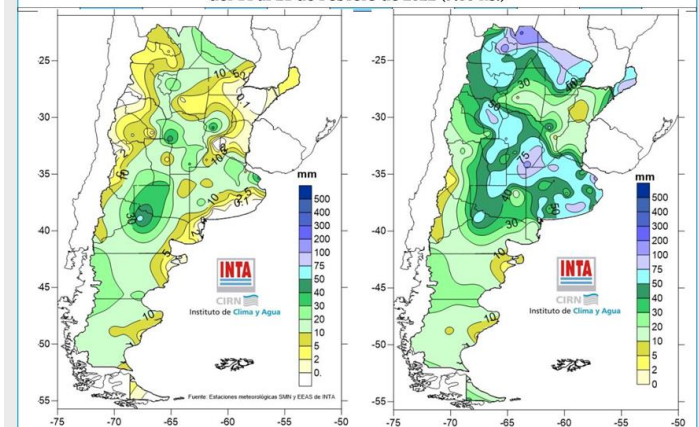
Fig. 01: Precipitación (mm) observada entre el 14 al 21 de Febrero de 2022 (9:00 hs.).
